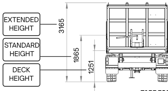
TARE 5600 GVM 1700
